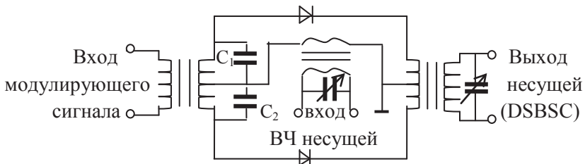
Рис. 1.3. Балансный модулятор: C1, C2 — конденсаторы развязки
