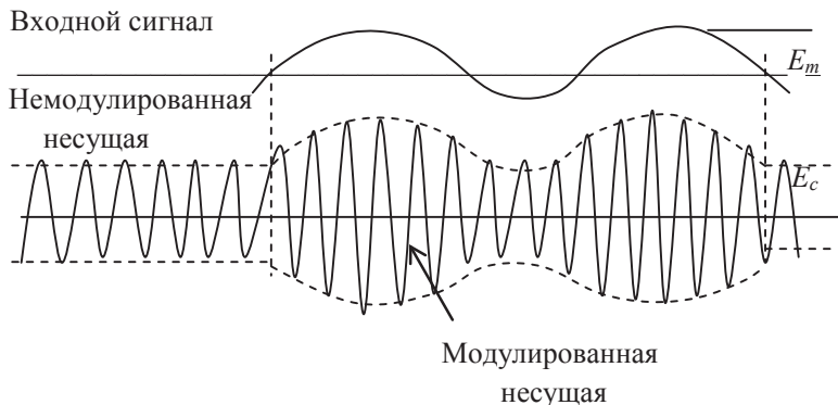
Рис. 1.1. Амплитудная модуляция
