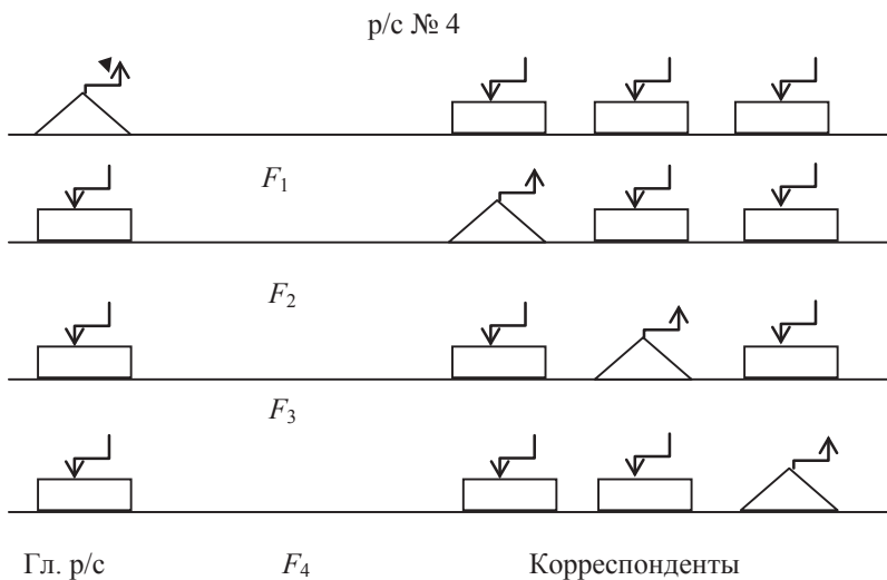
Рис. 7.6. Организация связи на частотах передатчиков
